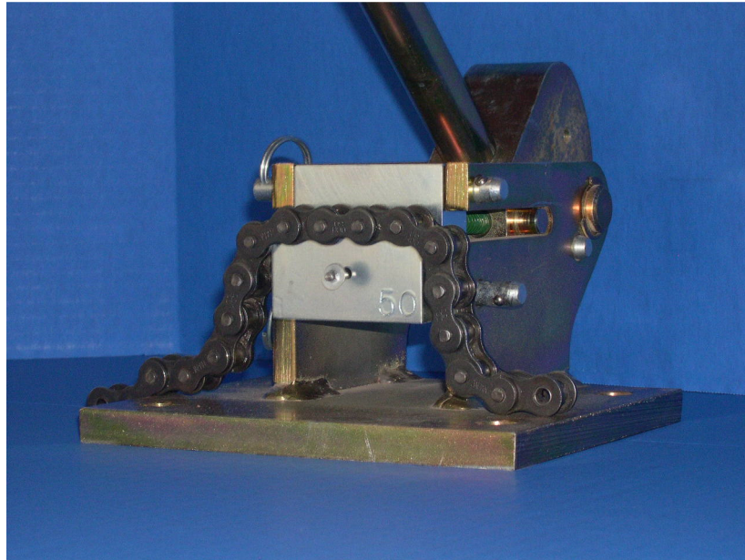
EZ_Breaker Basis-Einheit mit Werkzeug
