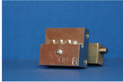
Trennwerkzeug 08B
